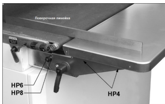
Рис. 5-4: выравнивание удлинения стола
