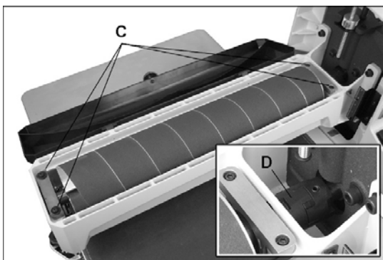
Рис. 9-2: извлечение барабана
